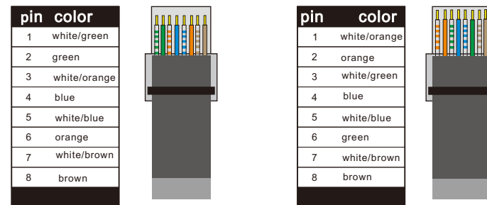
EIA/TIA 568A
